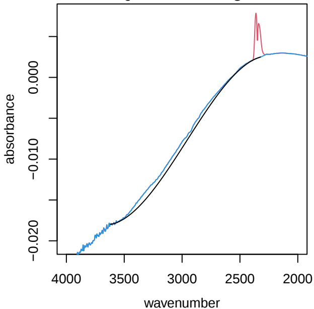
UTQ334 alkane region
