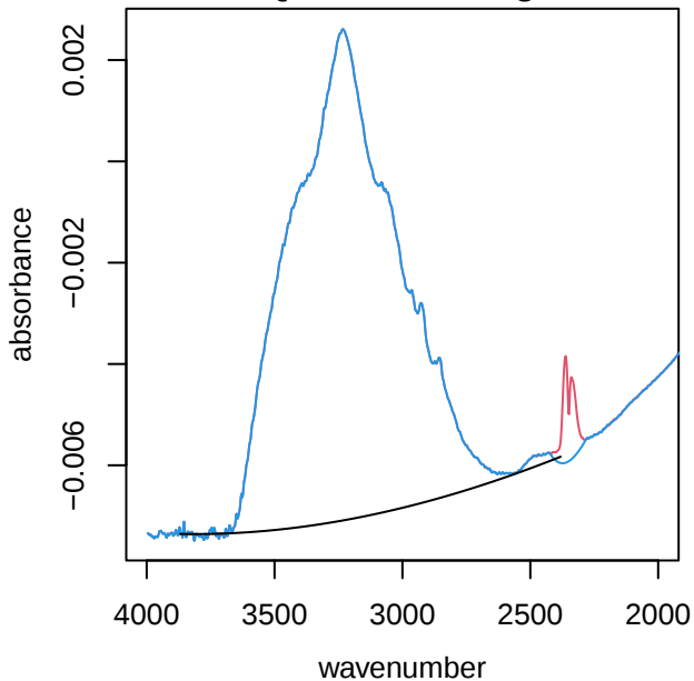
UTQ308 alkane region
