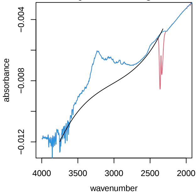
UTQ307 alkane region
