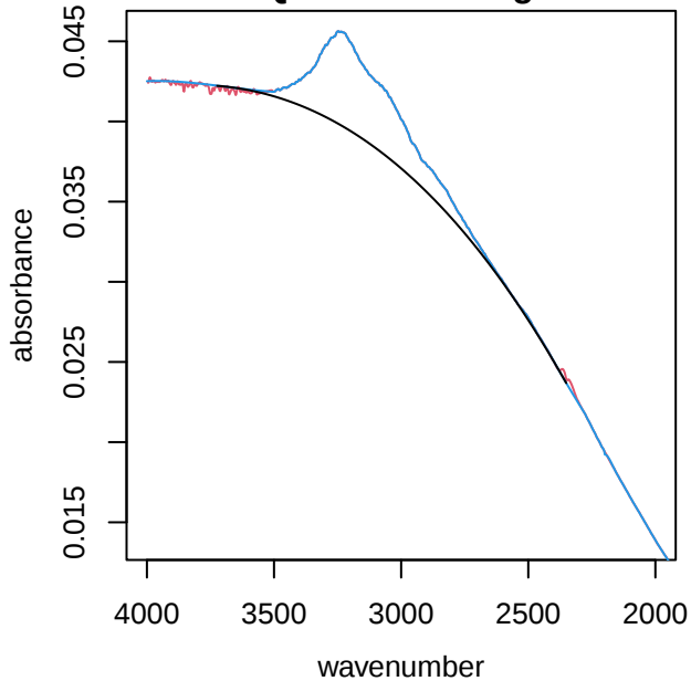
UTQ341 alkane region
