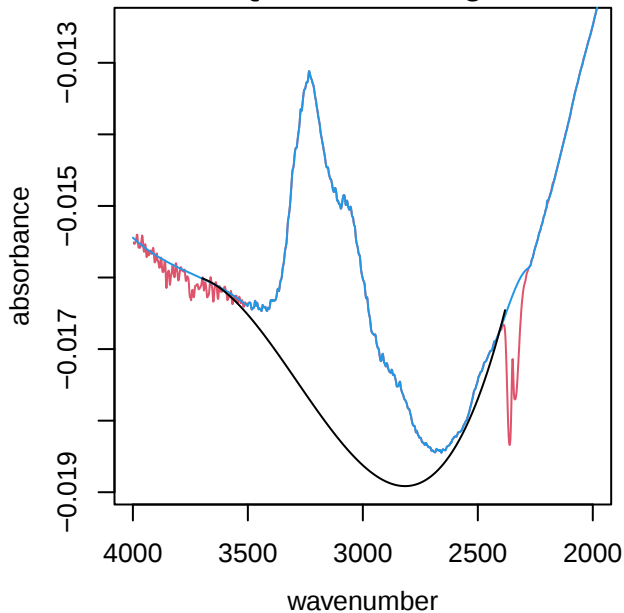
UTQ309 alkane region
