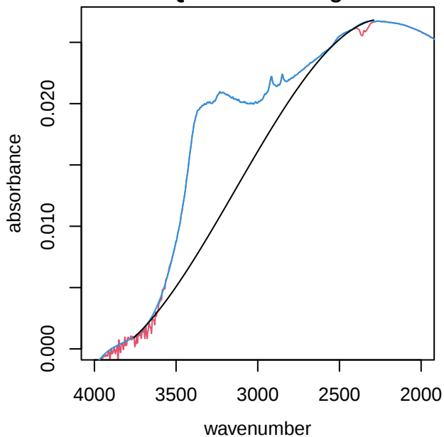
UTQ079 alkane region
