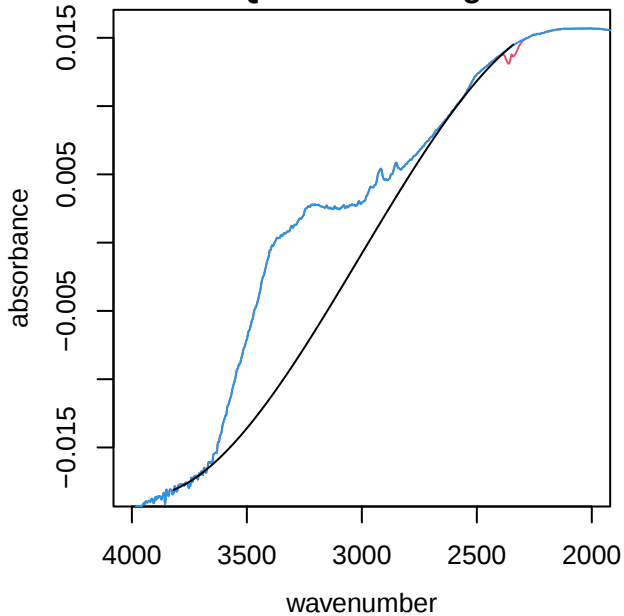
UTQ038 alkane region
