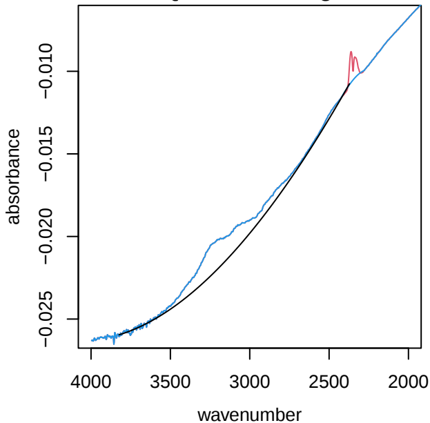
UTQ137 alkane region
