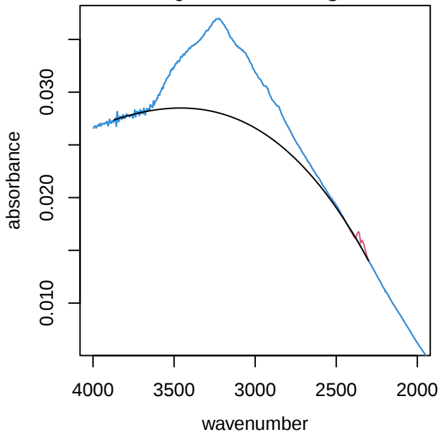
UTQ140 alkane region
