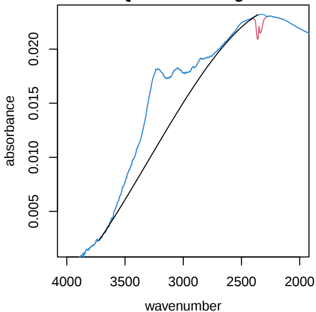
UTQ090 alkane region
