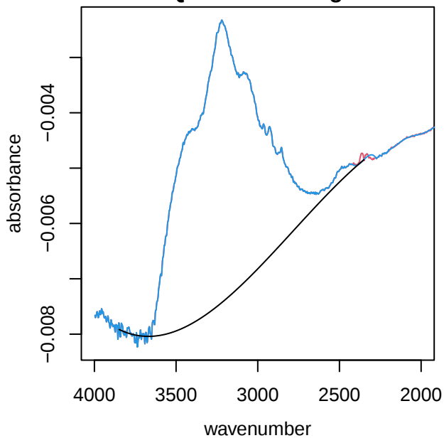
UTQ139 alkane region
