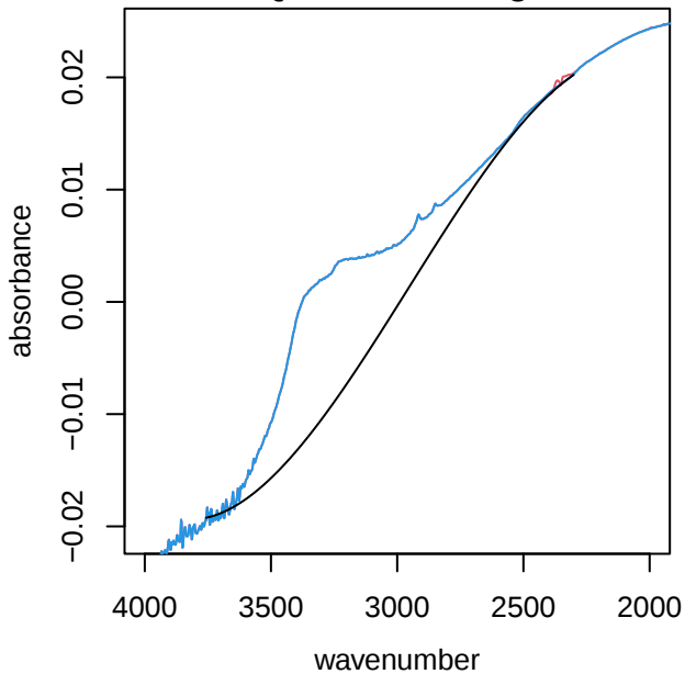
UTQ080 alkane region
