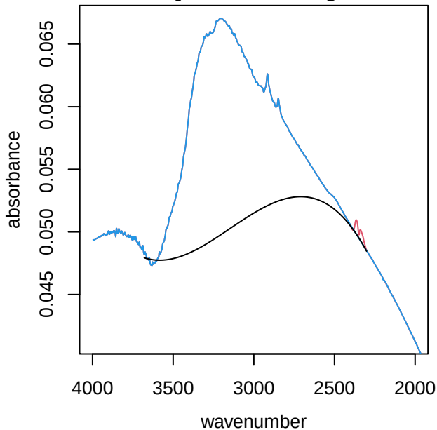
UTQ061 alkane region
