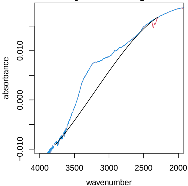
UTQ034 alkane region
