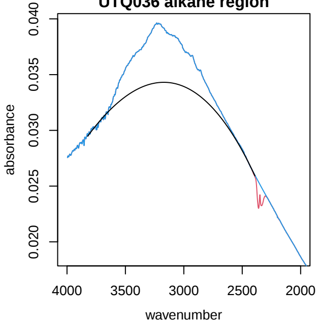
UTQ036 alkane region
