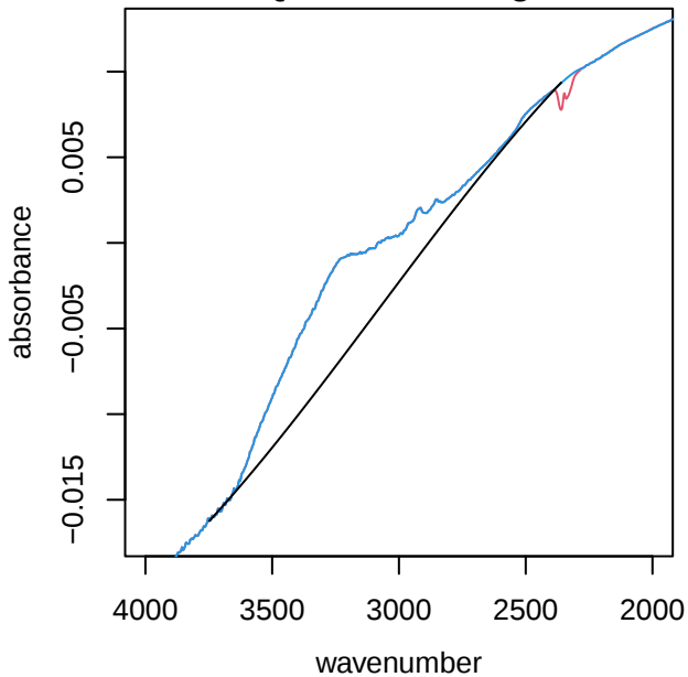
UTQ035 alkane region
