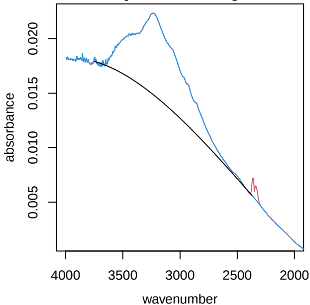
UTQ136 alkane region
