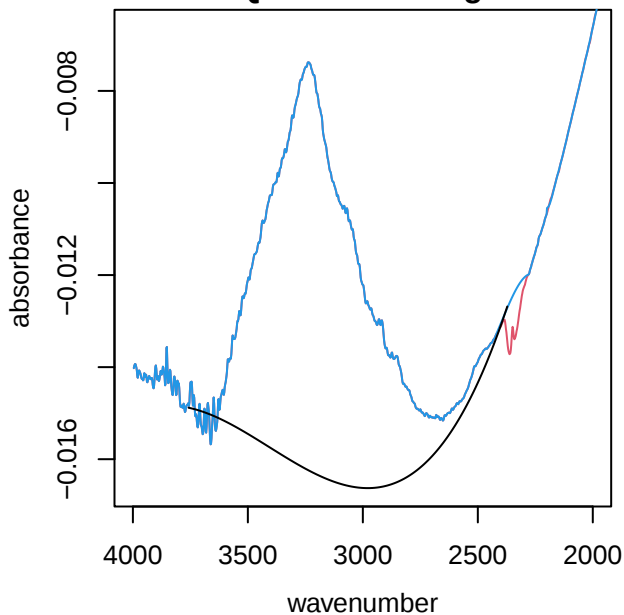
UTQ091 alkane region
