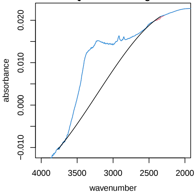
UTQ060 alkane region
