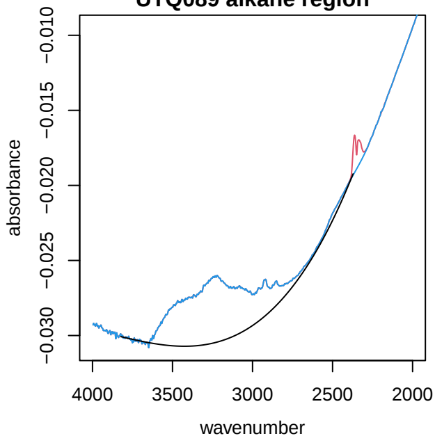
UTQ089 alkane region
