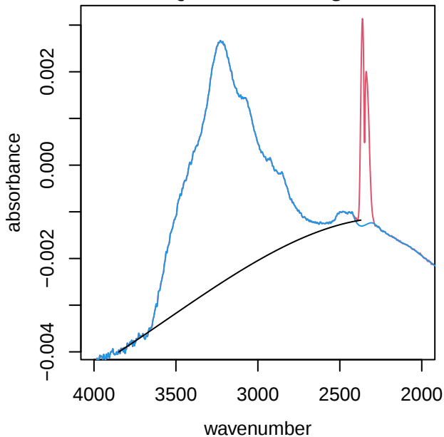
UTQ138 alkane region
