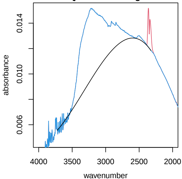
UTQ141 alkane region
