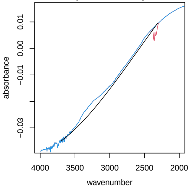
UTQ083 alkane region
