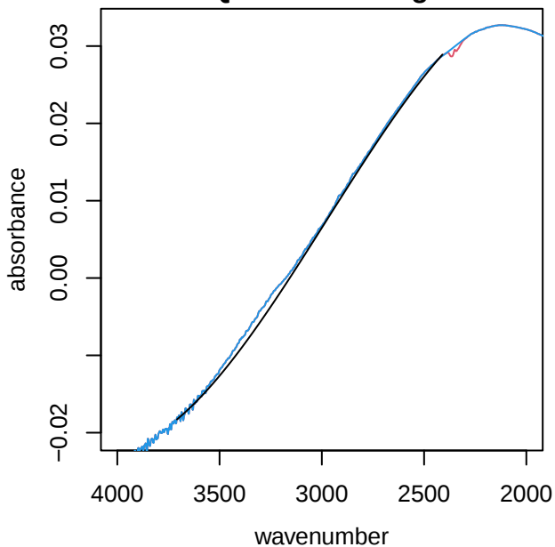
UTQ031 alkane region
