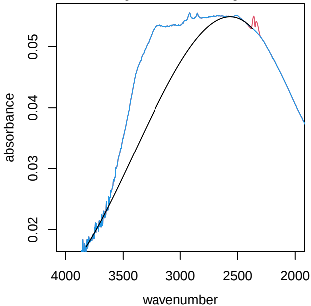
UTQ093 alkane region
