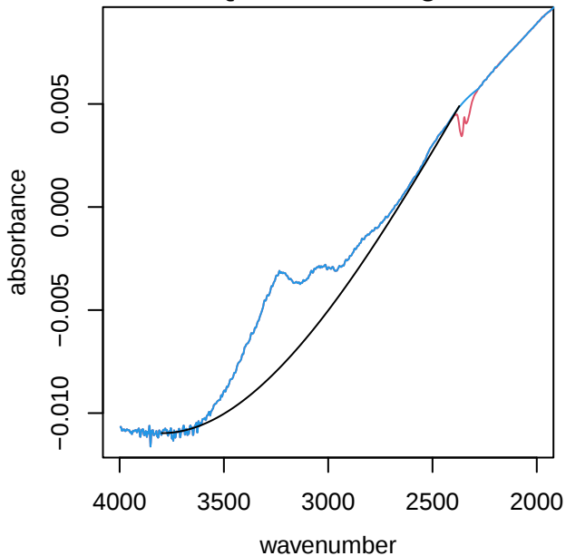
UTQ085 alkane region
