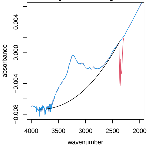
UTQ092 alkane region
