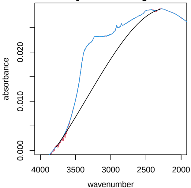
UTQ059 alkane region
