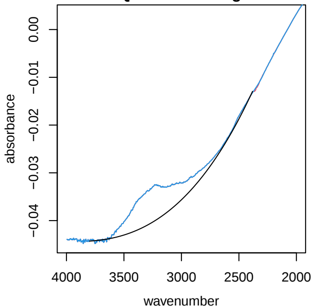
UTQ084 alkane region
