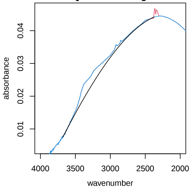
UTQ037 alkane region
