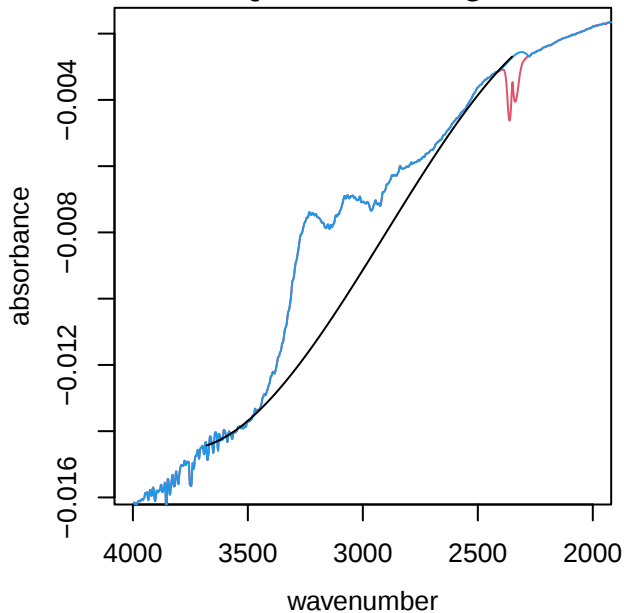
UTQ132 alkane region
