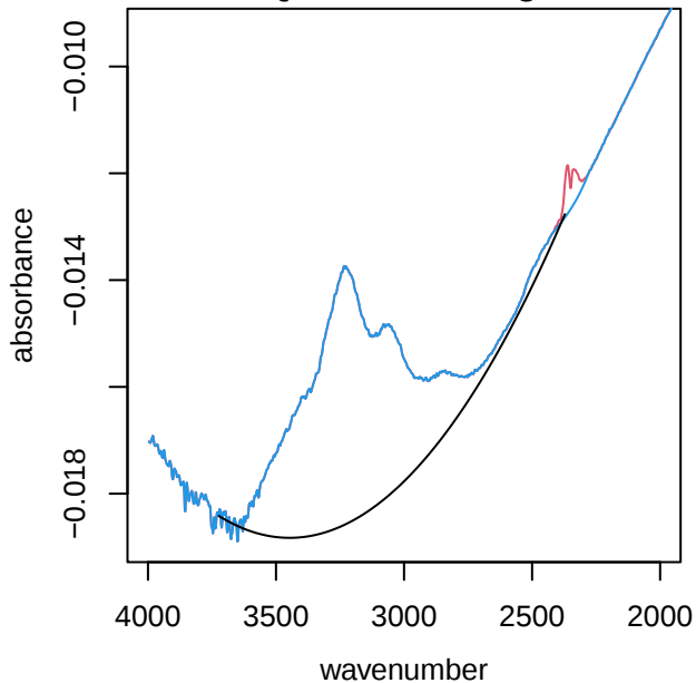
UTQ115 alkane region
