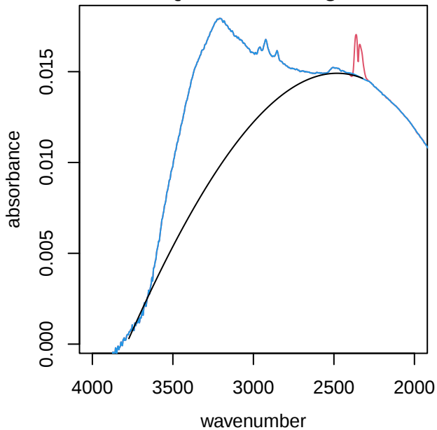
UTQ120 alkane region
