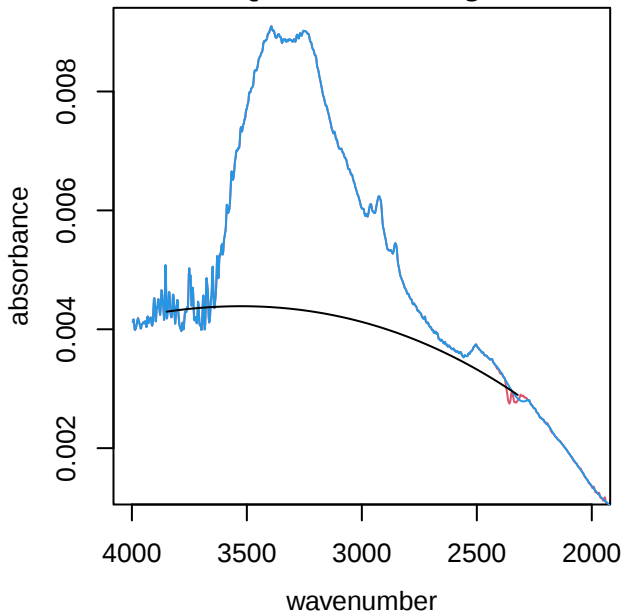
UTQ144 alkane region
