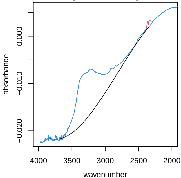
UTQ130 alkane region
