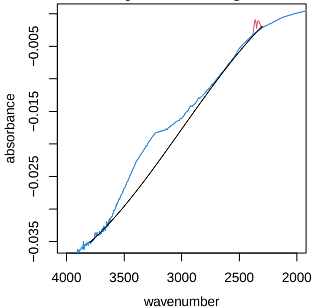
UTQ149 alkane region
