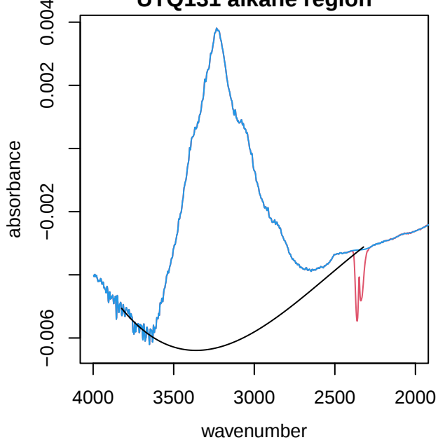
UTQ131 alkane region
