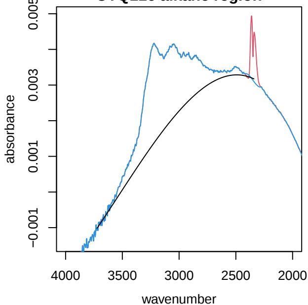
UTQ116 alkane region
