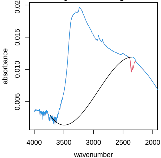
UTQ121 alkane region
