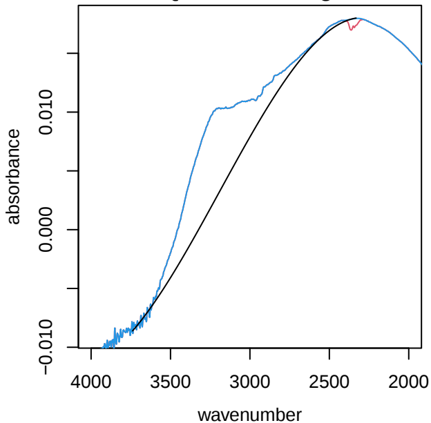
UTQ122 alkane region
