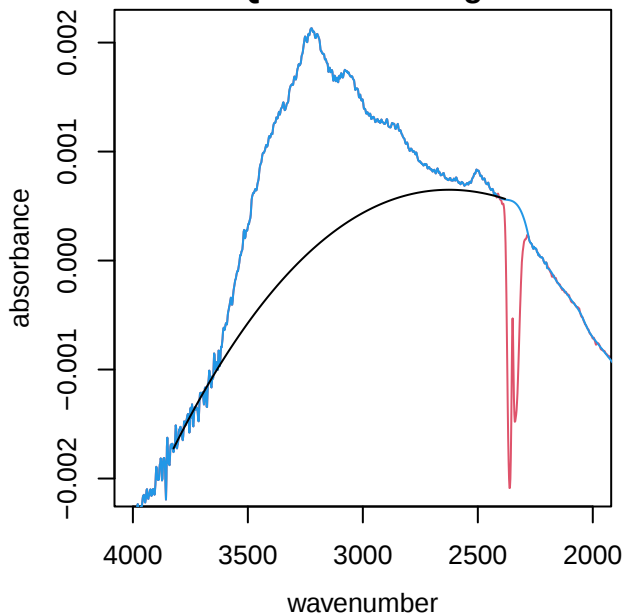
UTQ117 alkane region
