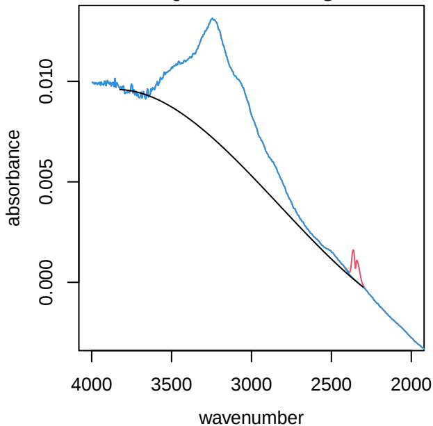
UTQ114 alkane region
