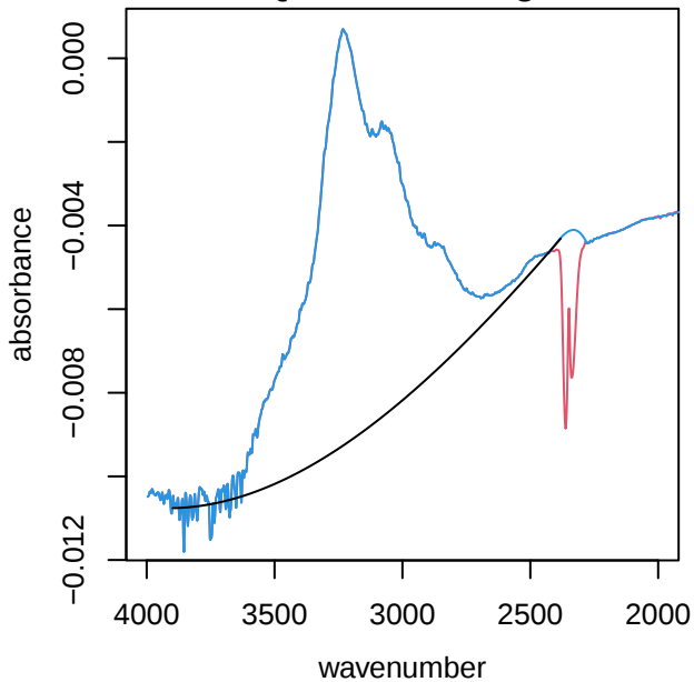
UTQ133 alkane region
