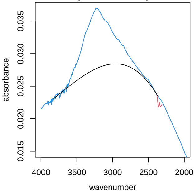
UTQ123 alkane region
