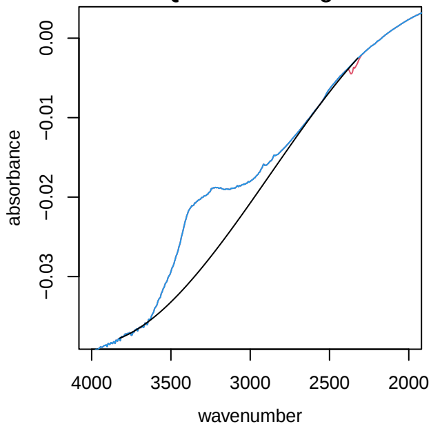
UTQ134 alkane region
