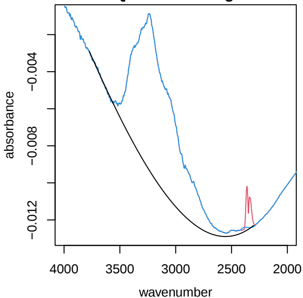
UTQ113 alkane region
