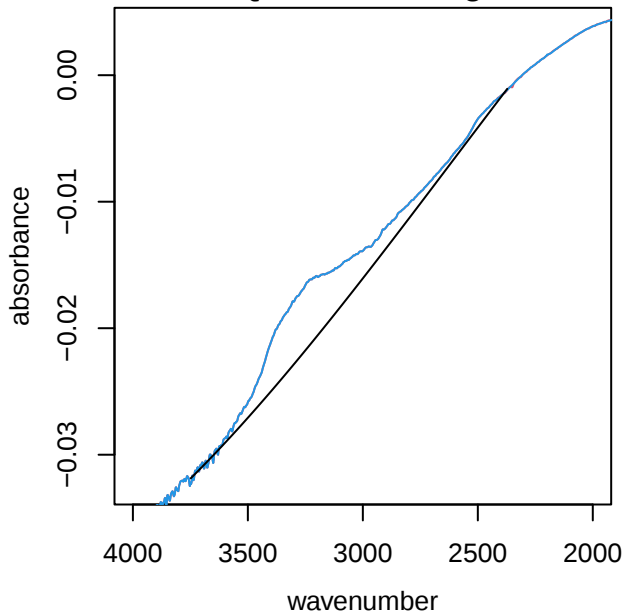
UTQ126 alkane region
