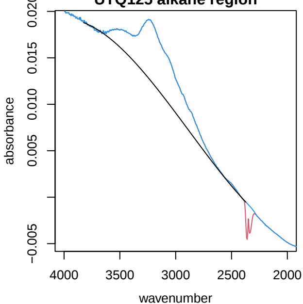
UTQ125 alkane region
