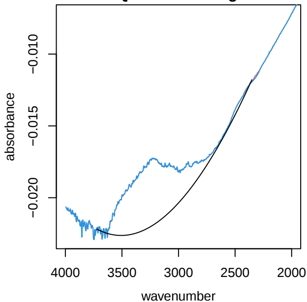
UTQ129 alkane region
