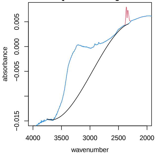
UTQ142 alkane region
