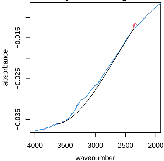
UTQ302 alkane region
