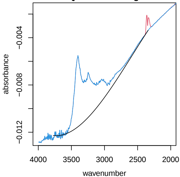
UTQ300 alkane region
