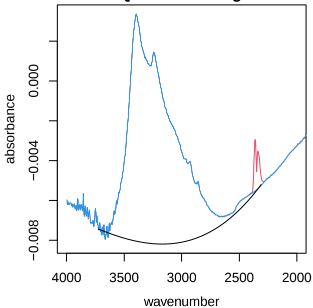
UTQ312 alkane region
