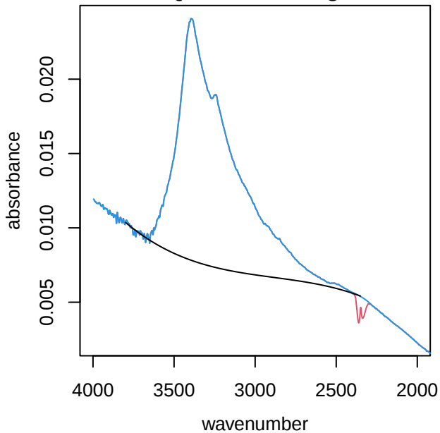
UTQ323 alkane region
