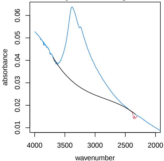
UTQ317 alkane region
