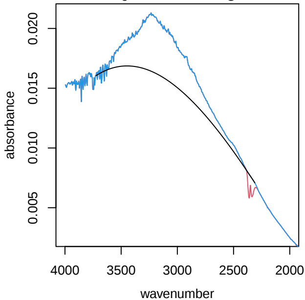
UTQ301 alkane region
