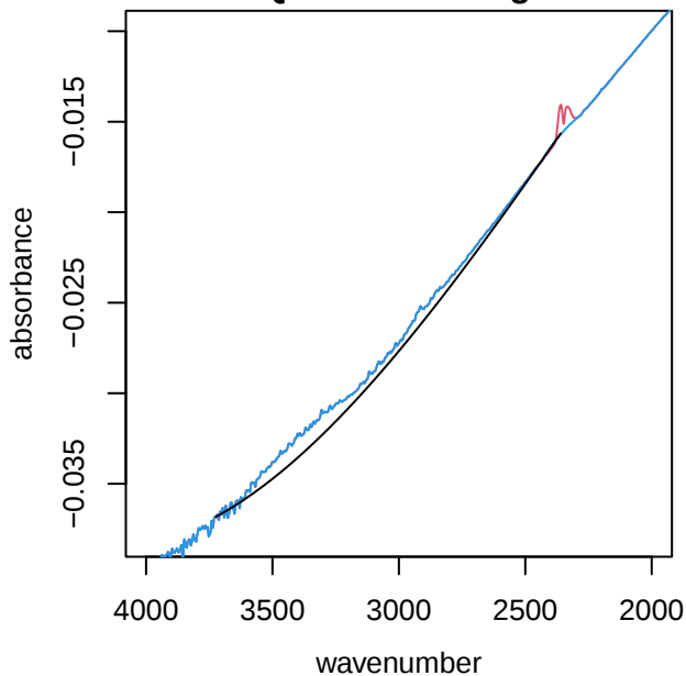
UTQ298 alkane region
