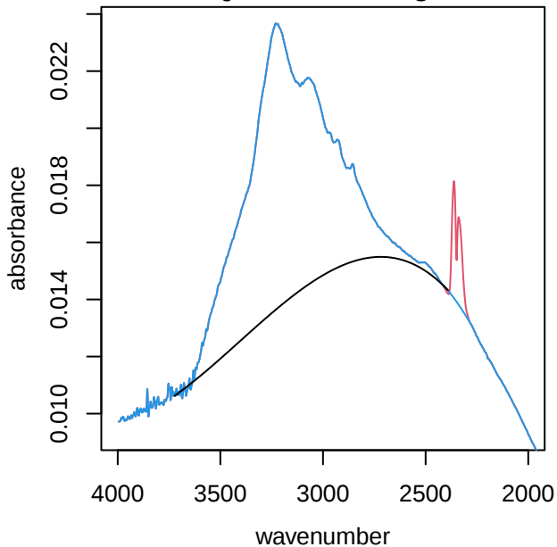
UTQ313 alkane region
