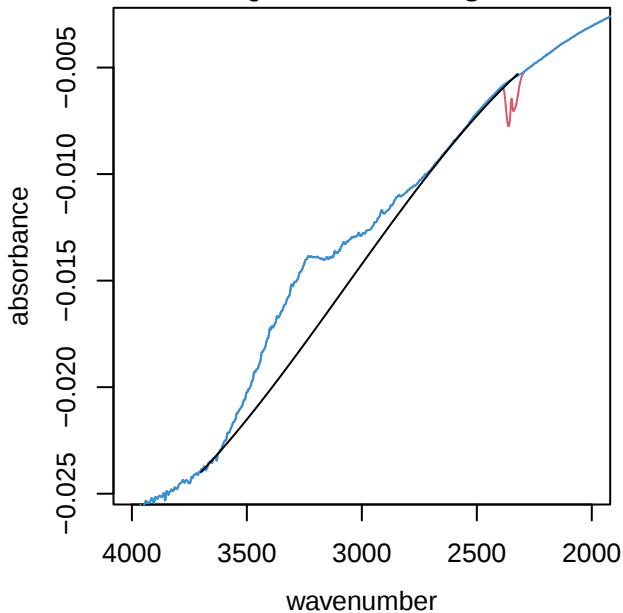
UTQ169 alkane region
