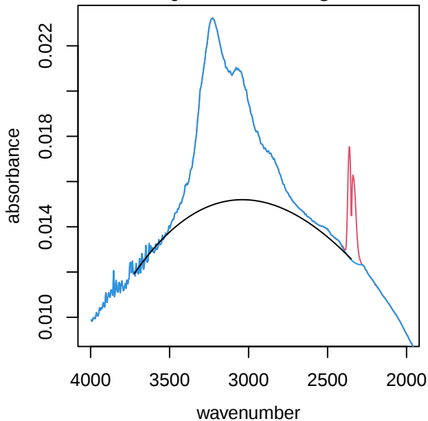
UTQ187 alkane region
