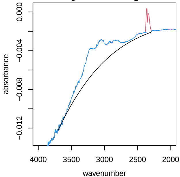
UTQ155 alkane region
