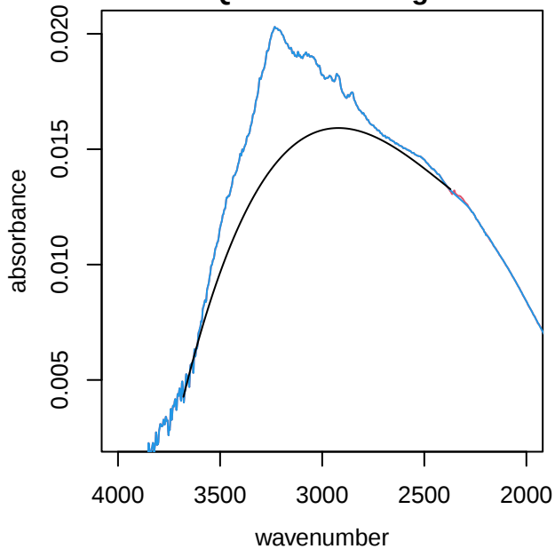
UTQ171 alkane region
