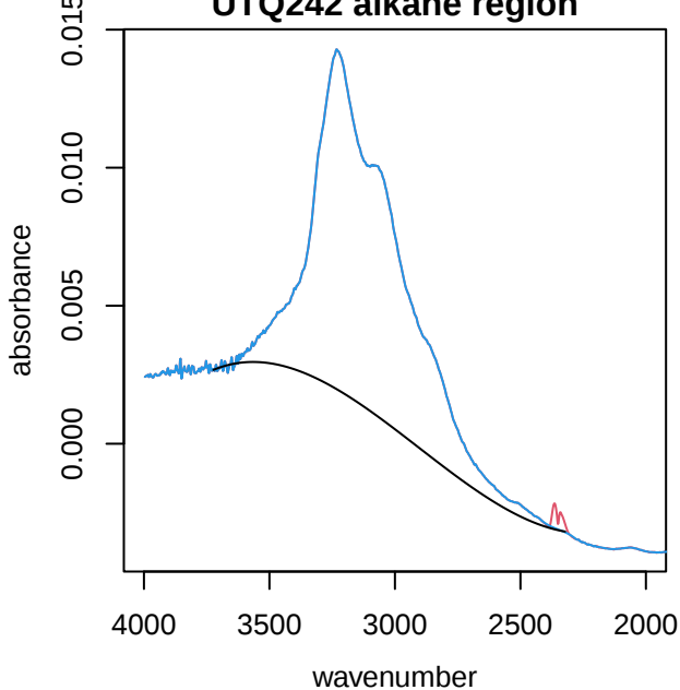
UTQ242 alkane region
