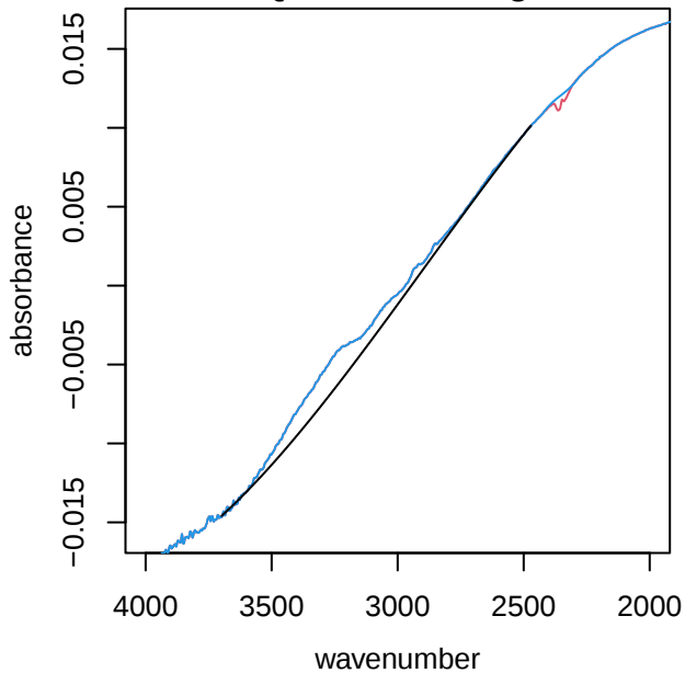
UTQ006 alkane region
