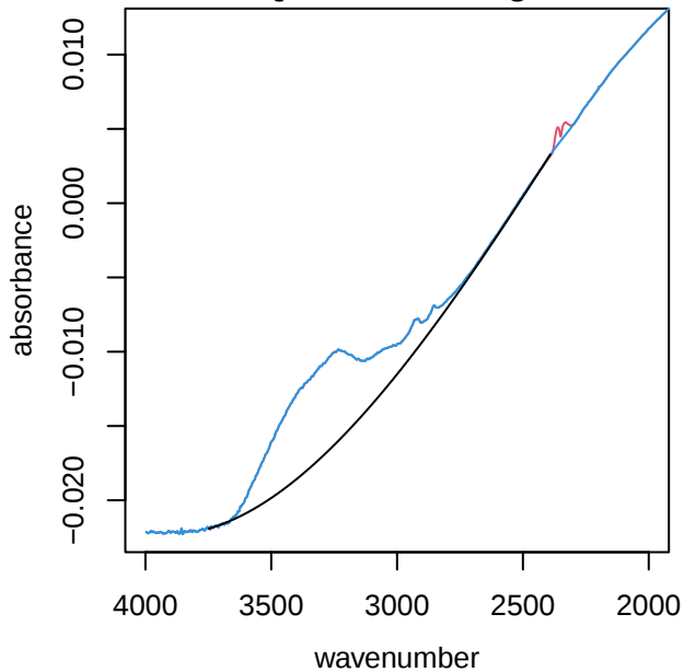
UTQ004 alkane region
