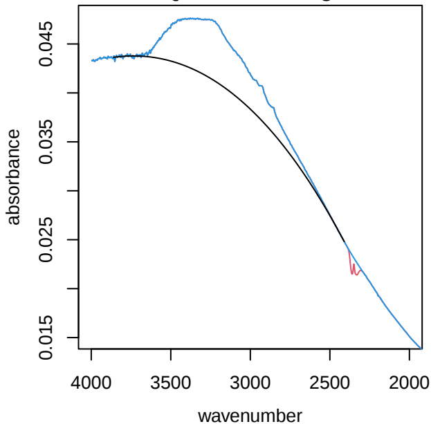
UTQ007 alkane region
