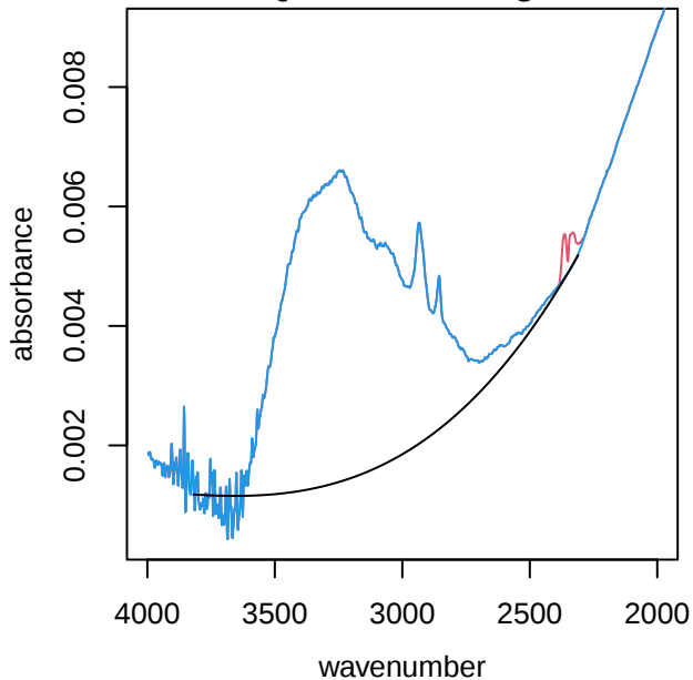
UTQ002 alkane region
