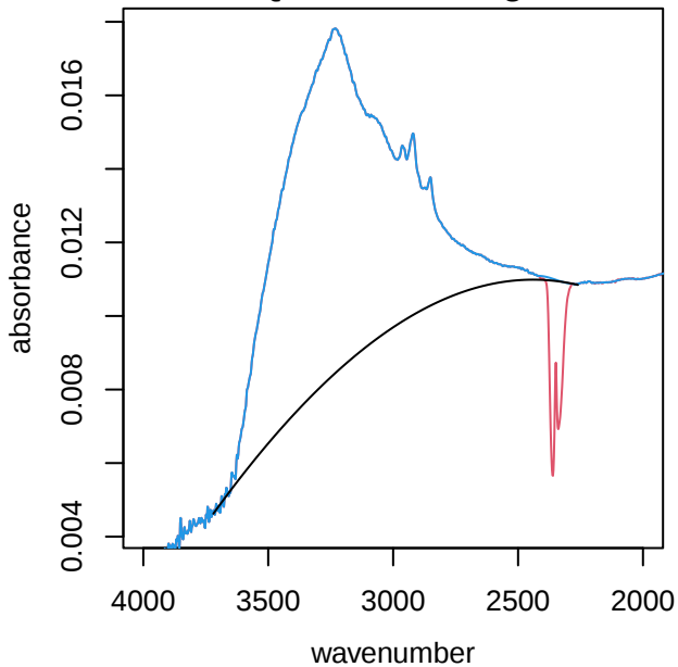
UTQ053 alkane region
