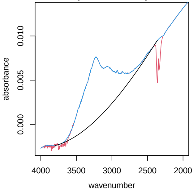
UTQ056 alkane region
