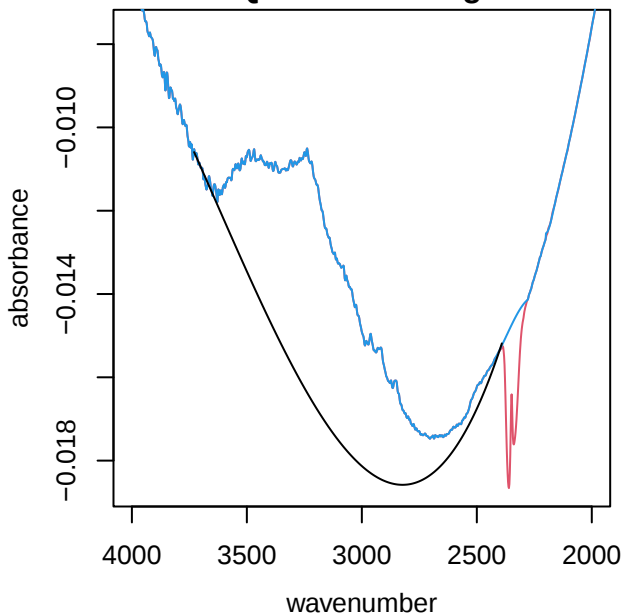
UTQ054 alkane region
