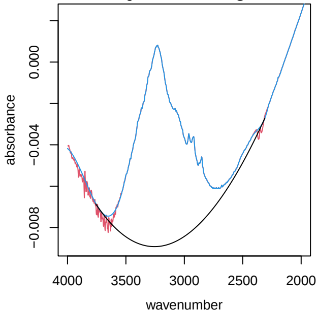
UTQ052 alkane region
