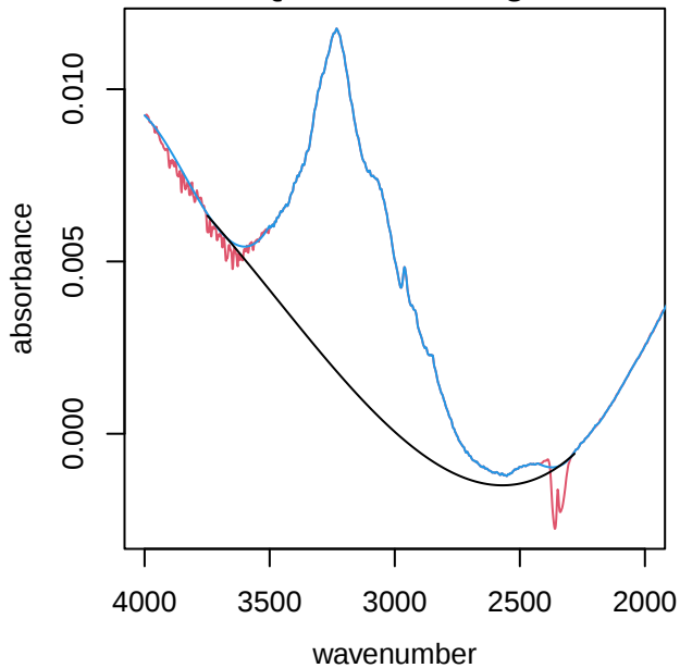
UTQ055 alkane region
