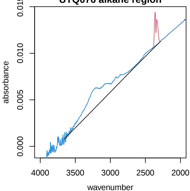
UTQ076 alkane region
