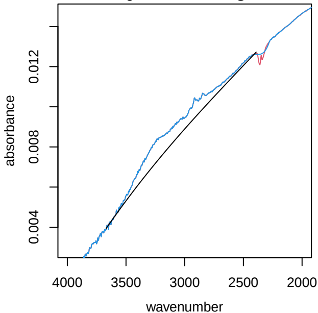
UTQ075 alkane region
