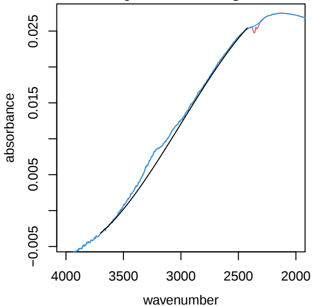
UTQ064 alkane region
