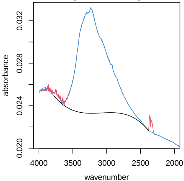
UTQ074 alkane region
