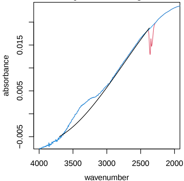
UTQ066 alkane region
