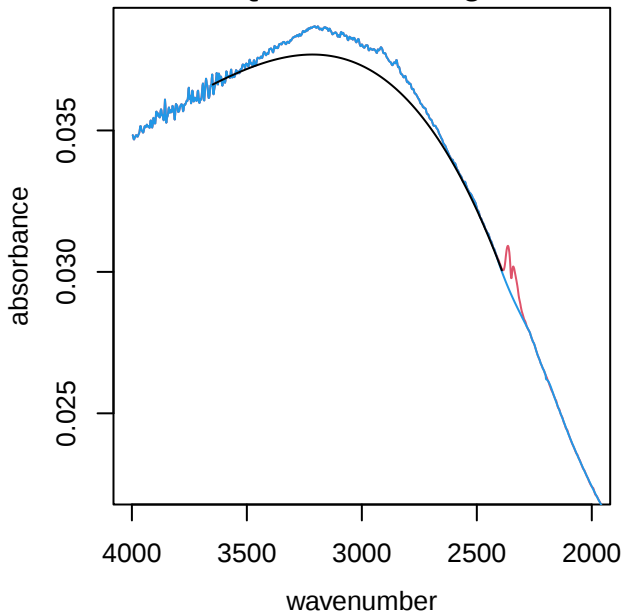
UTQ067 alkane region
