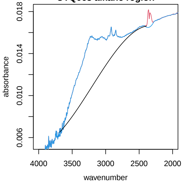
UTQ063 alkane region
