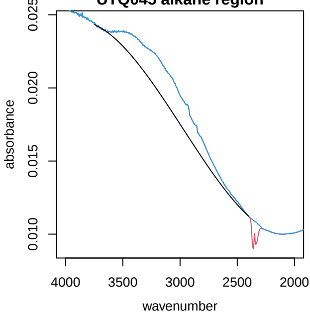
UTQ045 alkane region
