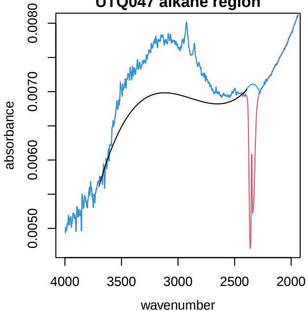
UTQ047 alkane region
