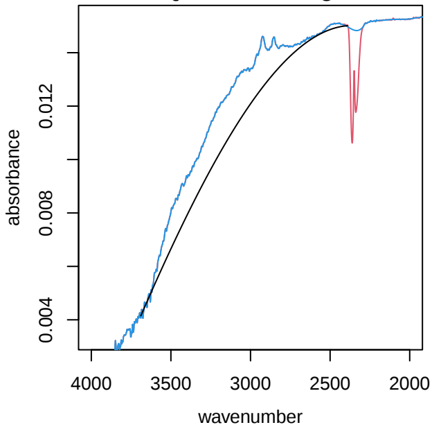
UTQ048 alkane region
