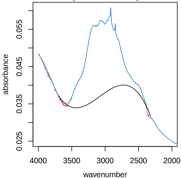
UTQ042 alkane region
