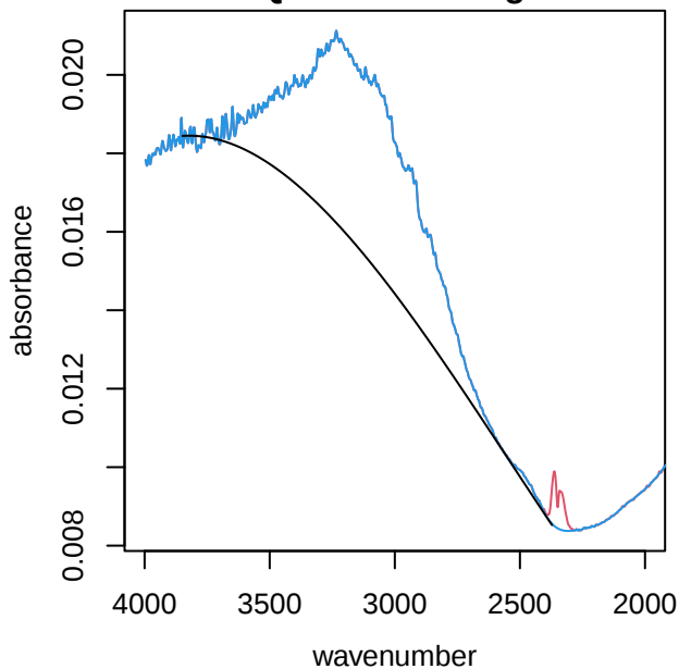
UTQ044 alkane region
