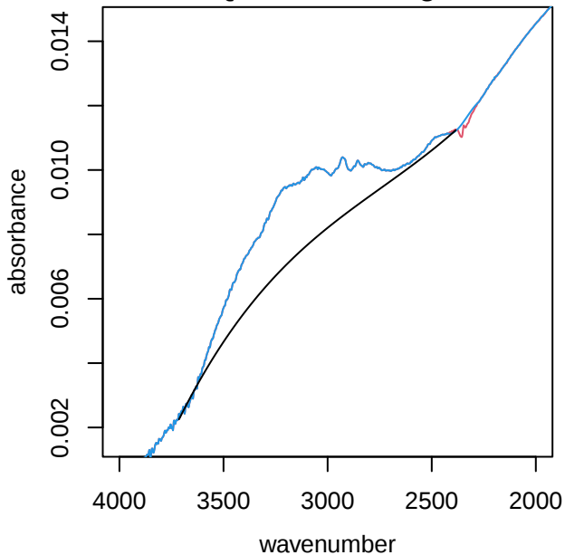
UTQ046 alkane region
