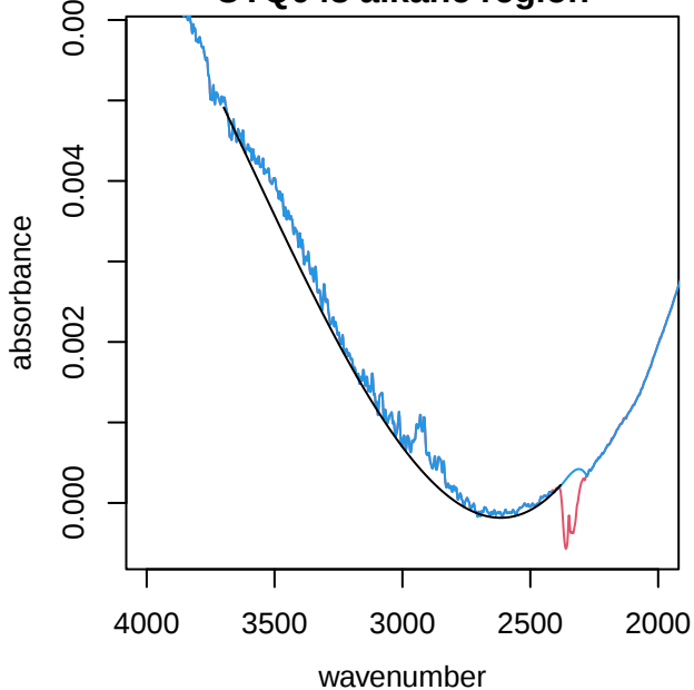
UTQ043 alkane region
