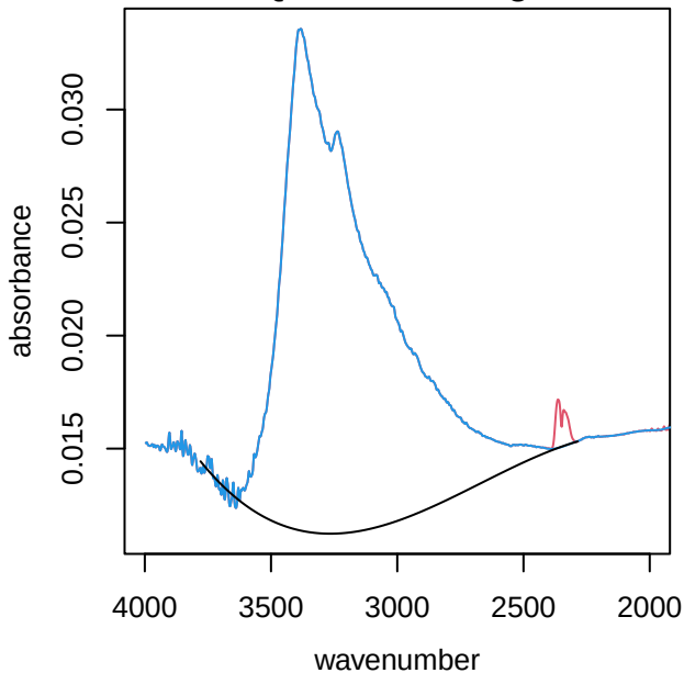
UTQ030 alkane region
