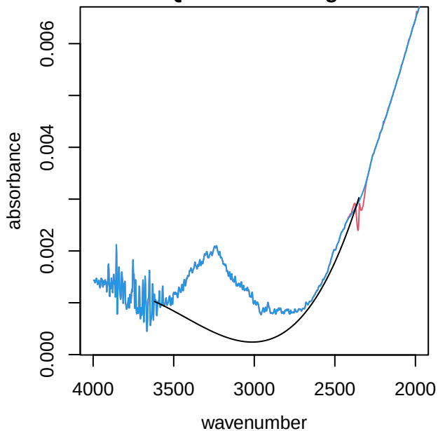
UTQ101 alkane region
