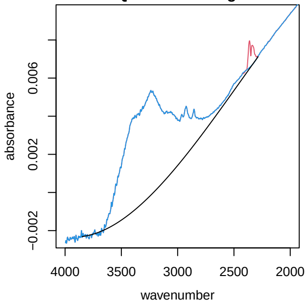
UTQ018 alkane region
