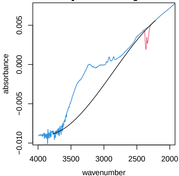
UTQ019 alkane region
