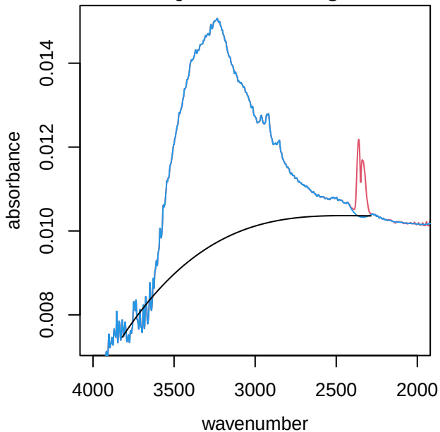
UTQ099 alkane region
