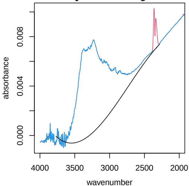
UTQ029 alkane region
