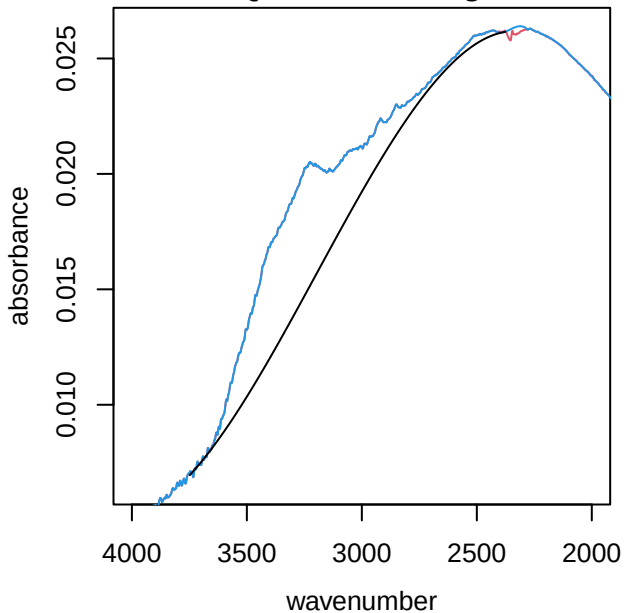
UTQ021 alkane region
