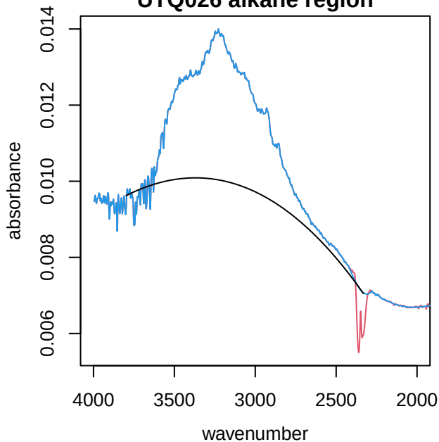
UTQ026 alkane region
