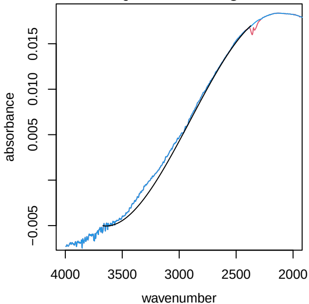
UTQ100 alkane region
