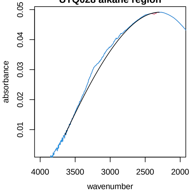
UTQ028 alkane region
