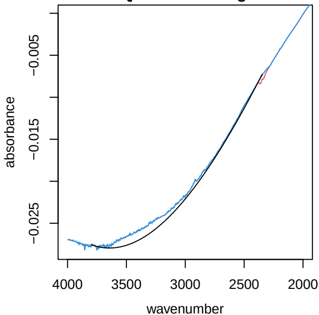
UTQ027 alkane region
