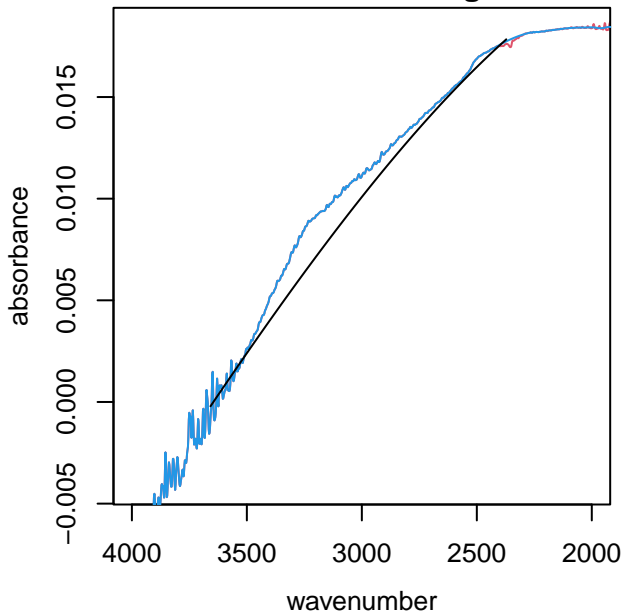
UTQ106 alkane region
