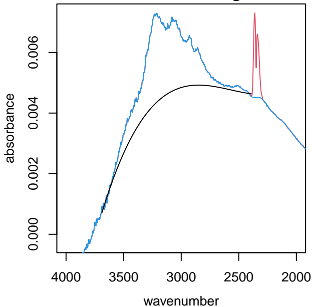
UTQ185 alkane region
