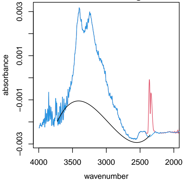
UTQ108 alkane region
