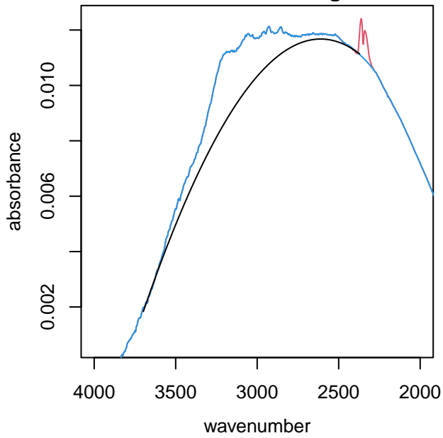
UTQ181 alkane region
