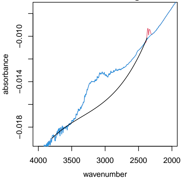
UTQ178 alkane region
