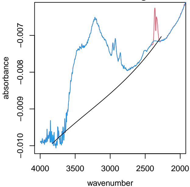
UTQ180 alkane region
