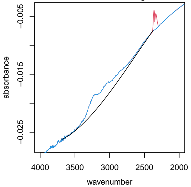
UTQ160 alkane region
