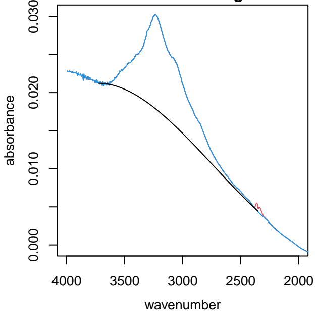
UTQ184 alkane region
