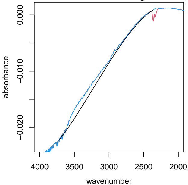
UTQ177 alkane region
