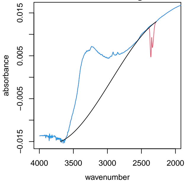
UTQ105 alkane region
