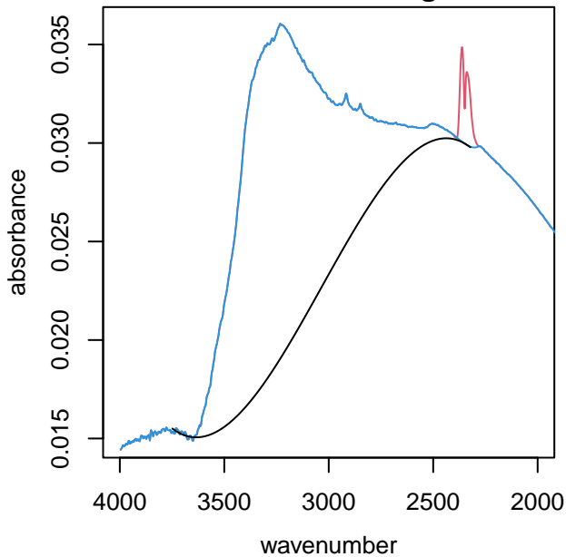
UTQ104 alkane region
