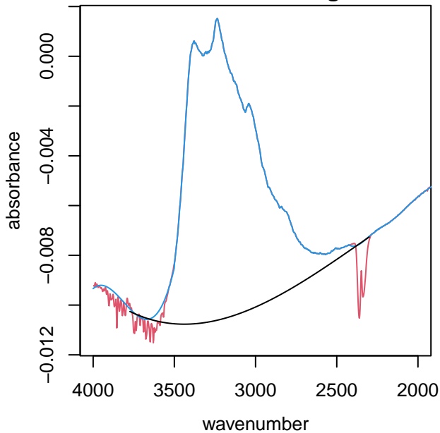
UTQ150 alkane region
