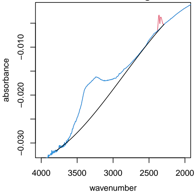
UTQ107 alkane region
